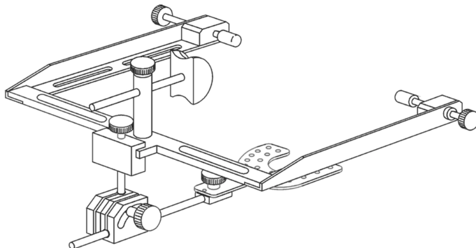
Abb. zeigt Gesichtsbogen ARTI S4 komplett Art.Nr.: 4207-001
